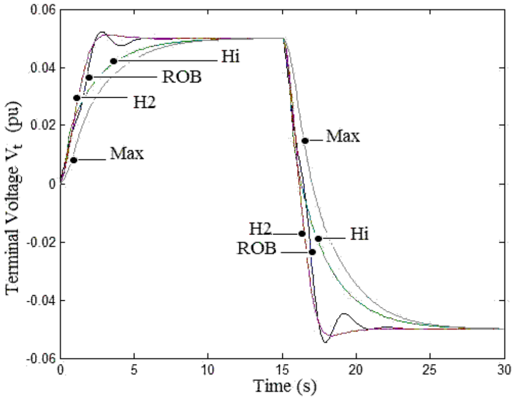
(d) Terminal voltage V_t
