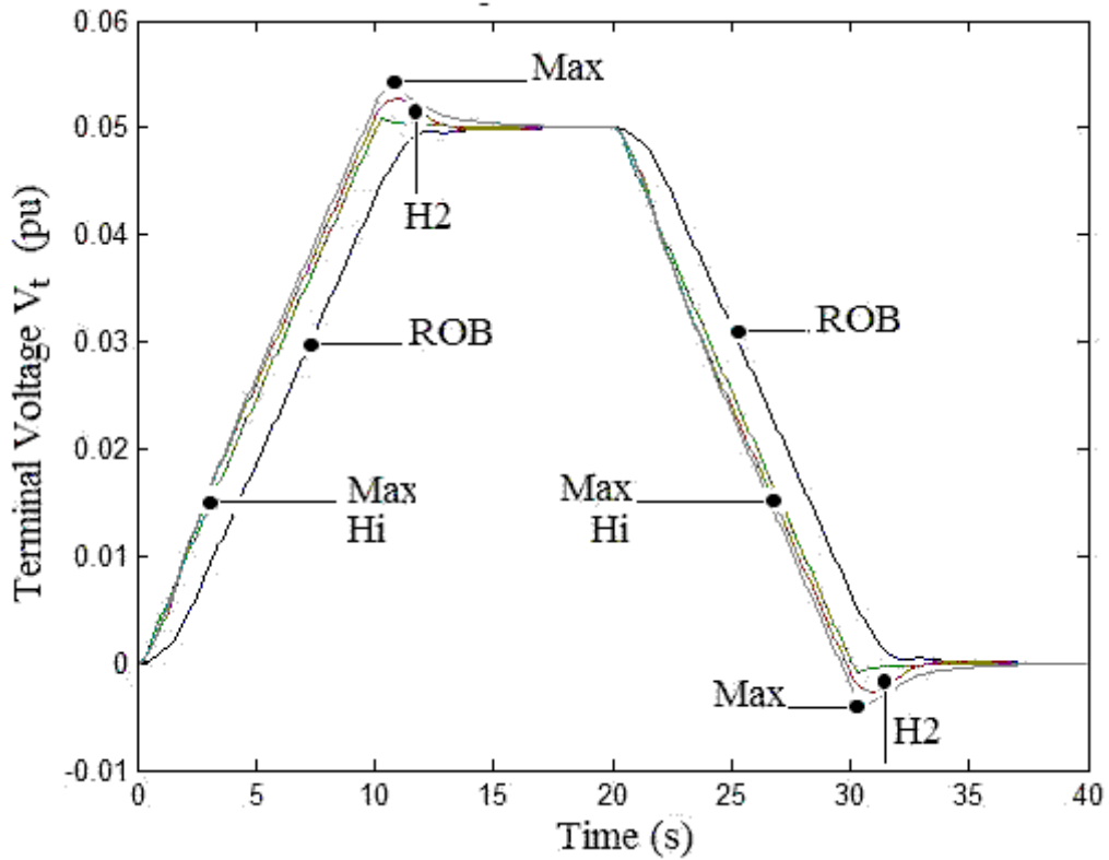
(d) Terminal voltage V_t
